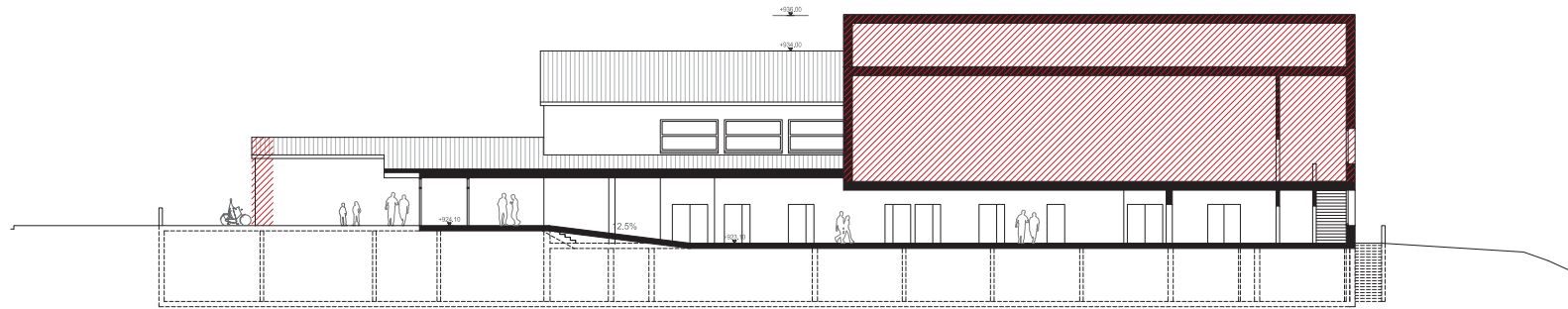
Schnitt A-A
